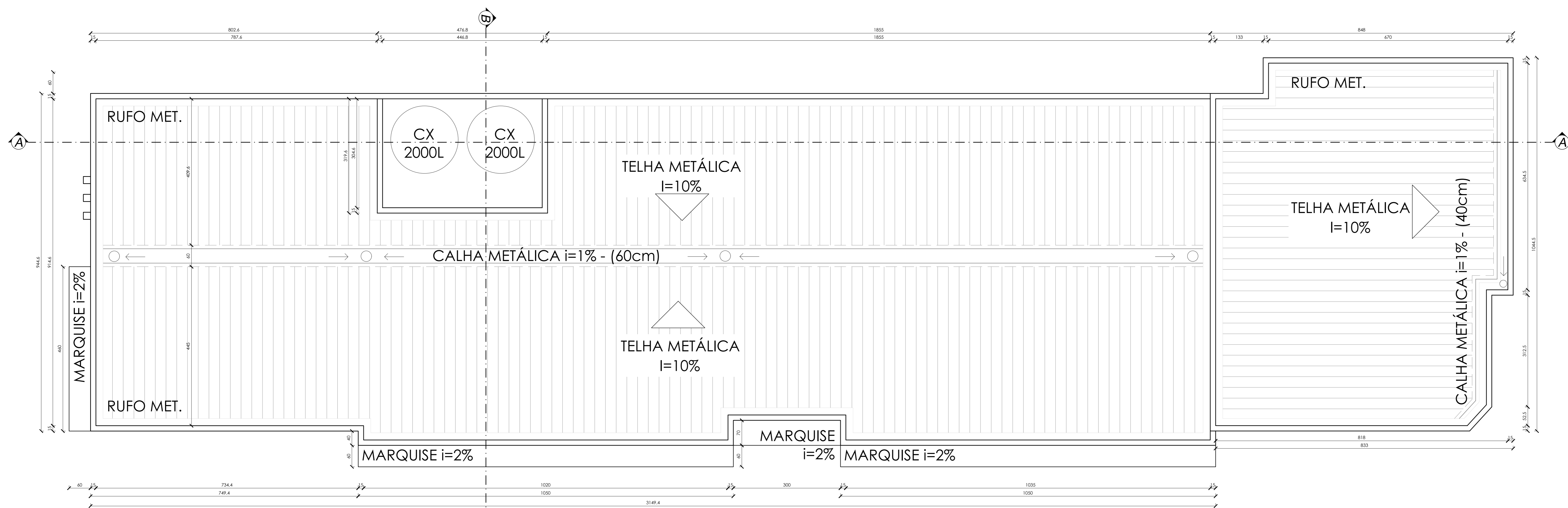
PLANTA DE COBERTURA ESC.: 1/50 ÁREA: 390,95m²
