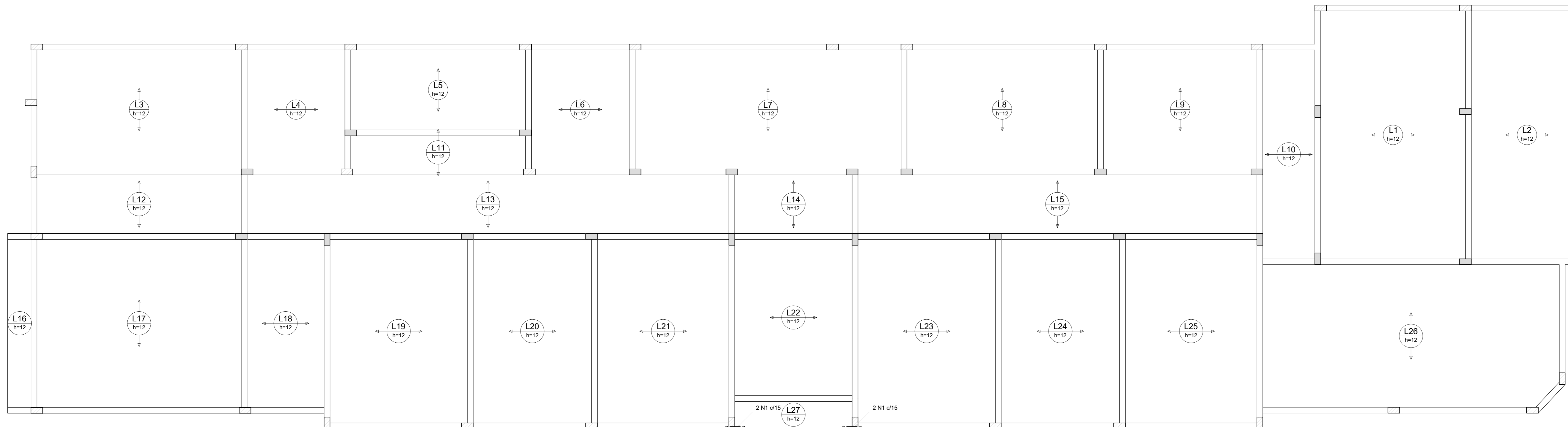
Armação negativa das lajes do pavimento COBERTURA (Eixo X)
