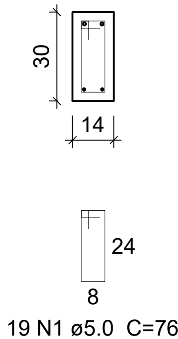
SEÇÃO A-A ESC 1:25
