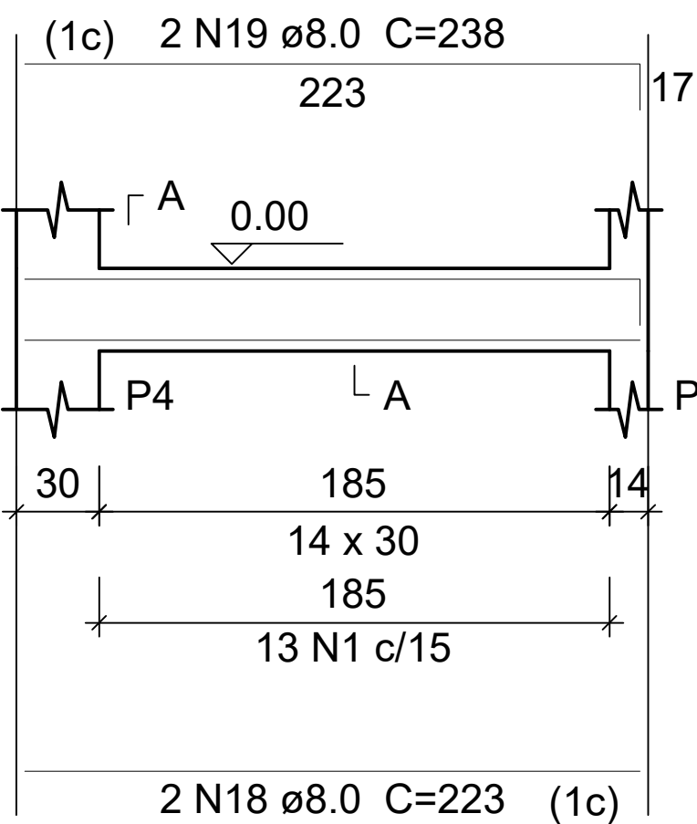
SEÇÃO A-A ESC 1:25
