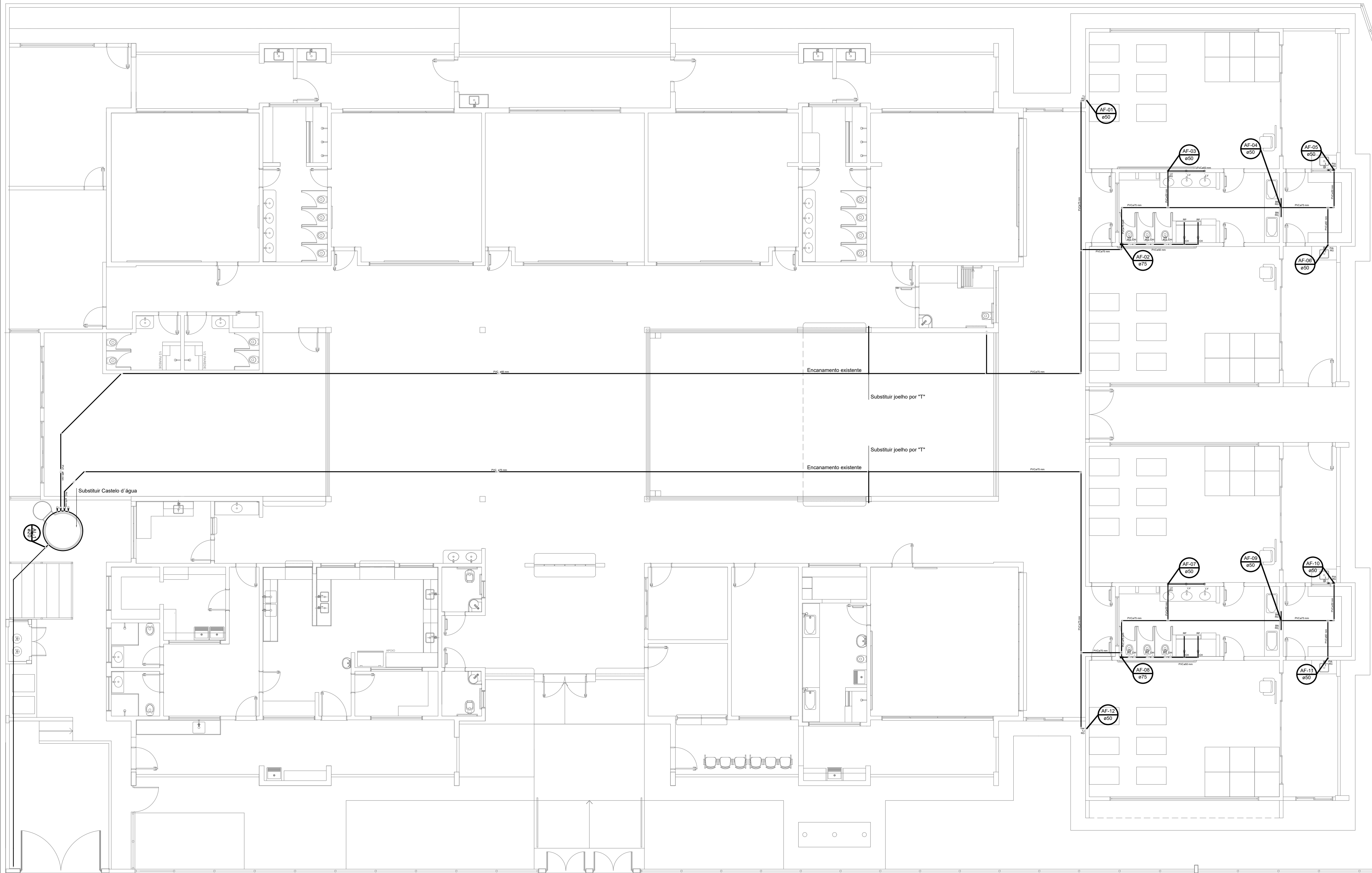
PLANTA ÁGUA FRIA ESC.:1/50
