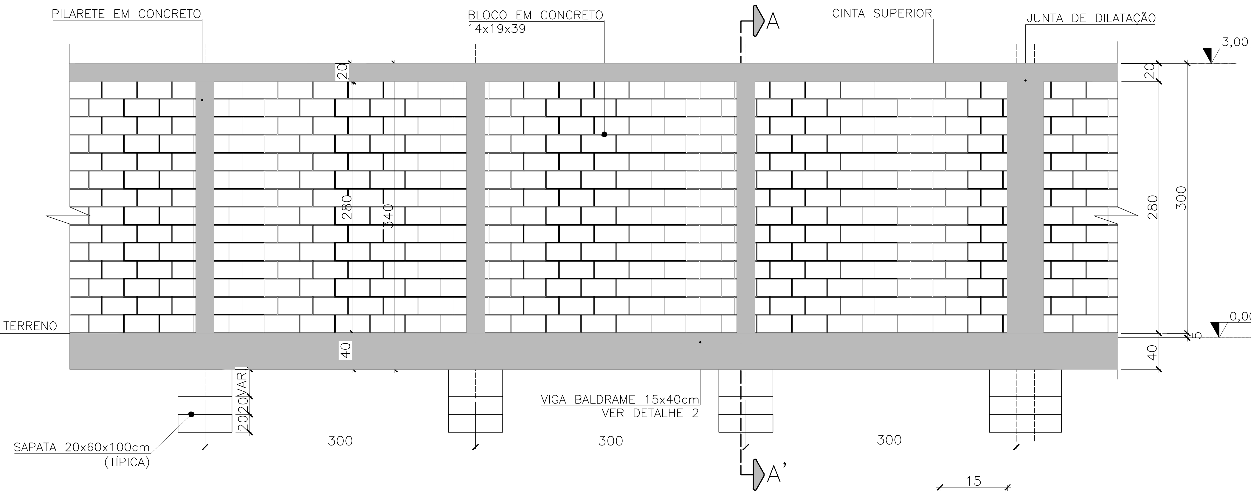
VISTA FRONTAL ESCALA: 1/50
