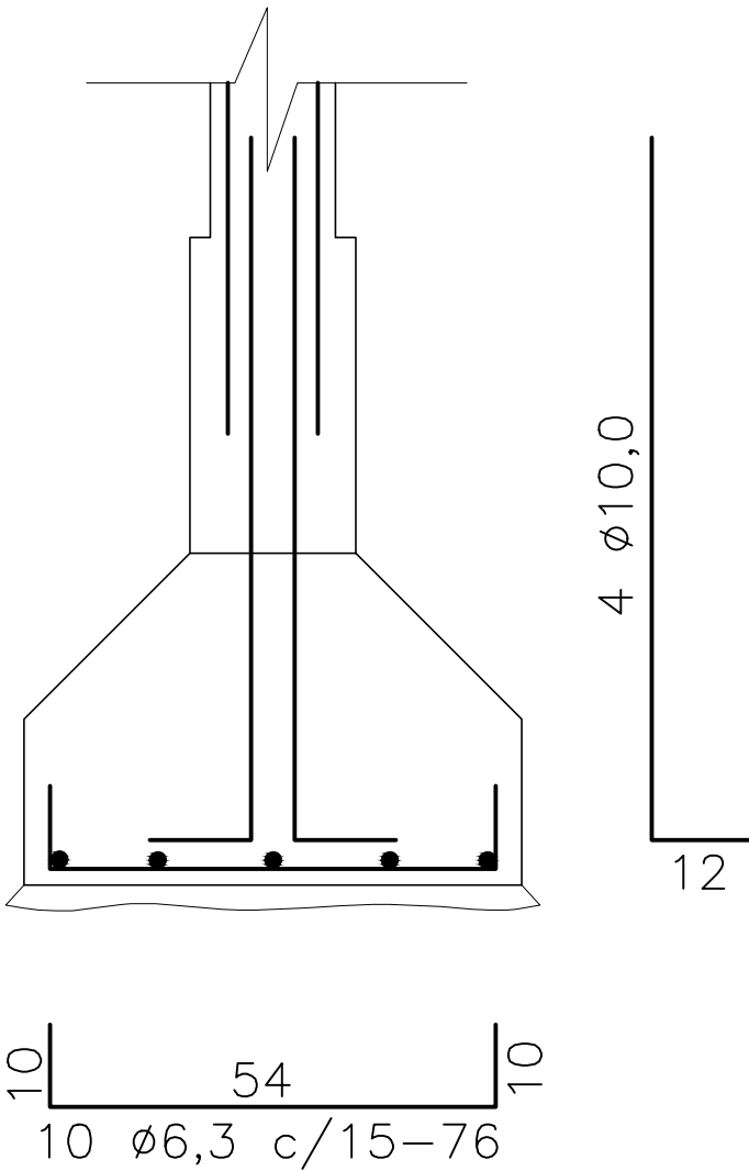
DETALHE SAPATA FERRAGENS ESCALA: 1/20
