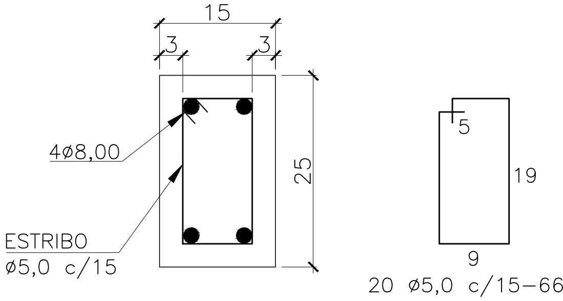
SEÇÃO DO PILAR ESCALA: 1/10
