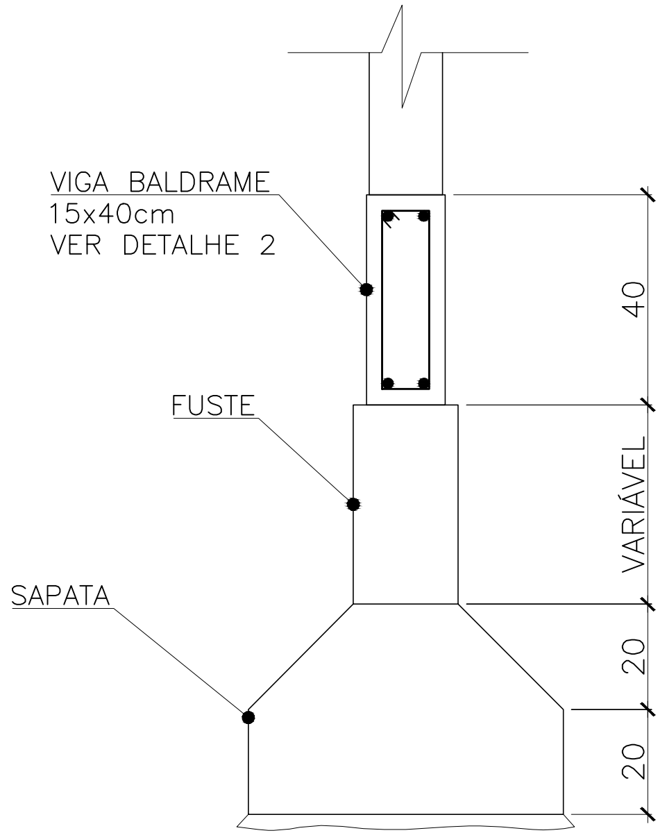
DETALHE TÍPICO SAPATA ESCALA: 1/20
