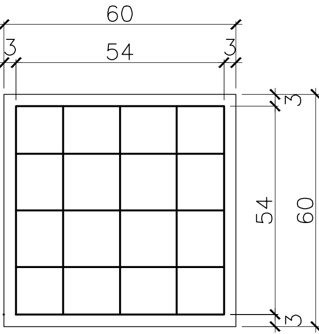
FUNDO DA SAPATA FERRAGENS ESCALA: 1/20
