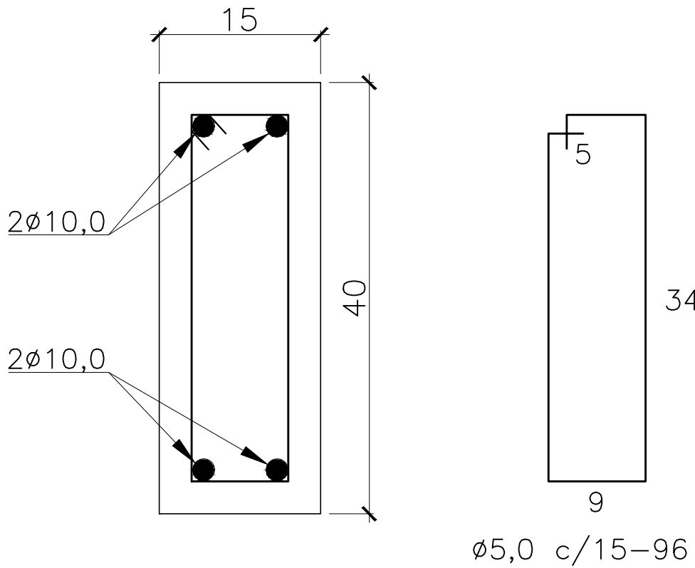
DETALHE 2 SEÇÃO VIGA BALDRAME ESCALA: 1/10
