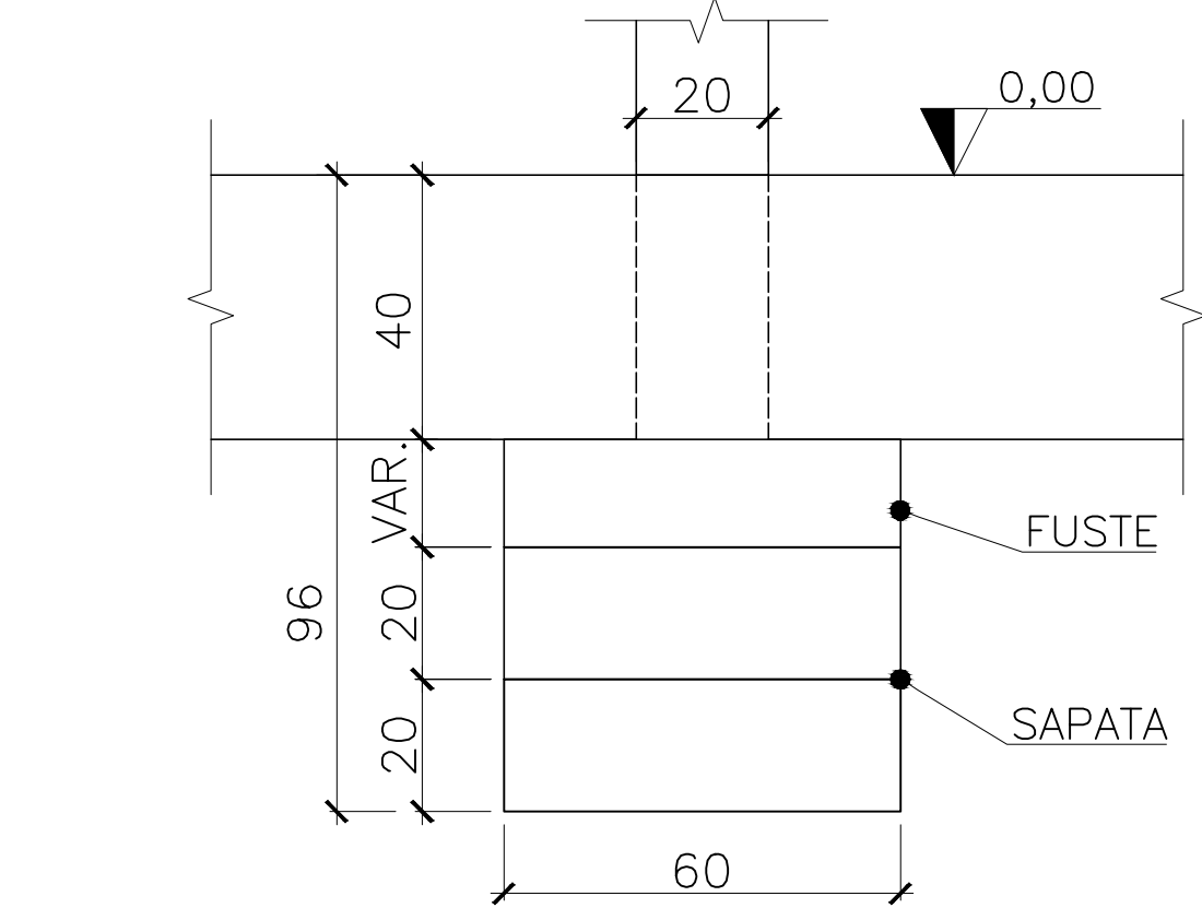
VIGA BALDRAME / SAPATA FORMA E VISTA ESCALA: 1/25
