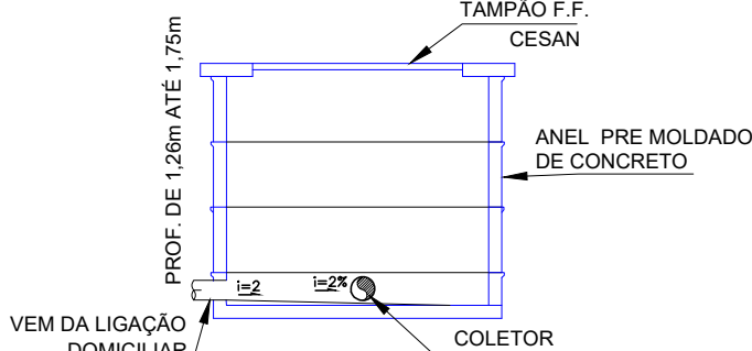
CORTE BB PV DN 1000 PROF. DE 1,26m ATÉ 1,75m SEM ESCALA
