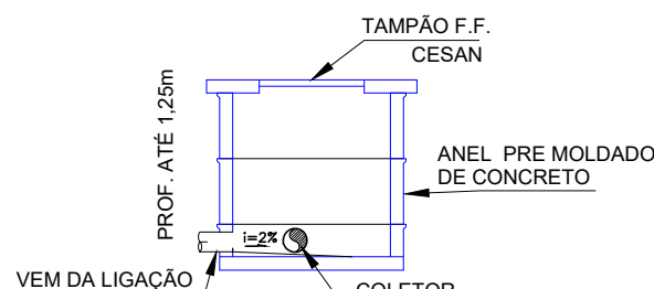
CORTE AA PV DN 600 PROF. ATÉ 1,25m SEM ESCALA
