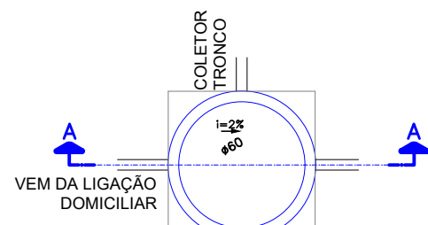
DETALHE 01 PV DN 600 SEM ESCALA
