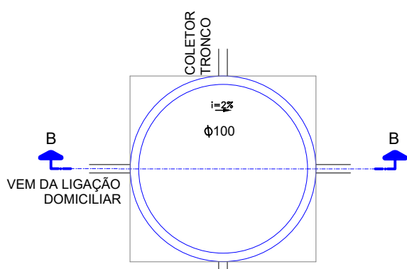
DETALHE 02 PV DN 1000 SEM ESCALA
