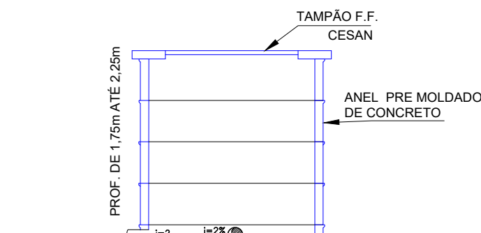
CORTE BB PV DN 1000 PROF. DE 1,75m ATÉ 2,25m SEM ESCALA
