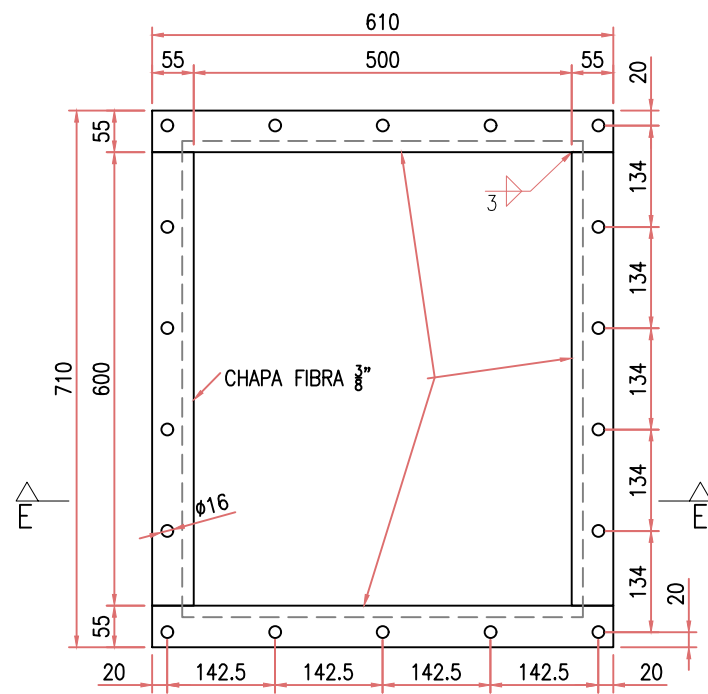
DETALHE 1 FL-VISTA SEM TAMPA (FLANGE) Escala: 1/10
