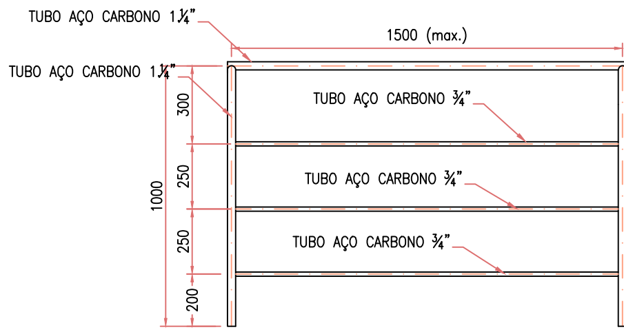
GUARDA CORPO PADRÃO DO TANQUE *TOTALMENTE REVESTIDO EM FIBRA Escala: 1/20
