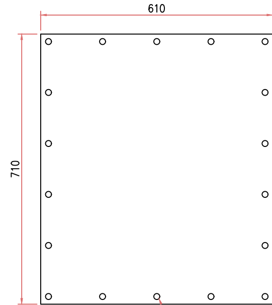
BORRACHA Lentil em Borracha 5MM Qtd.: 03 pçs. Escala: 1/10
