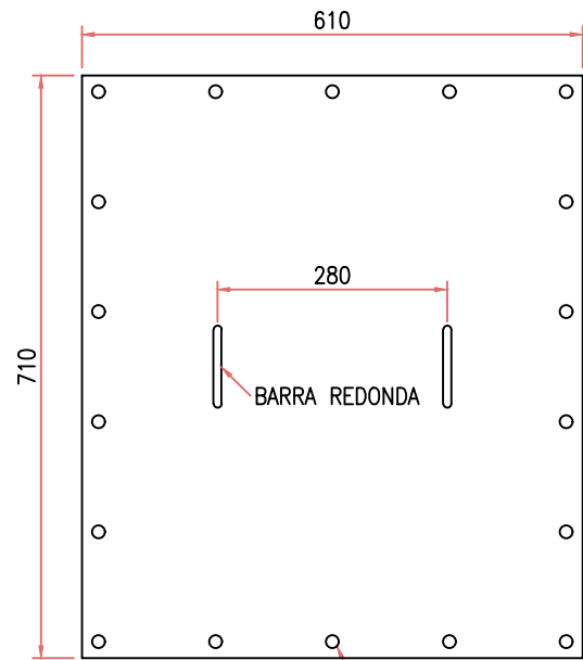
BOCA VISITA Chapa 3/8"x600x700 Qtd.: 07 pçs. Escala: 1/10
